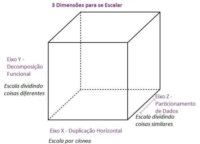
Fig. 2. Cubo Escala: modelo de escalabilidade em 3 dimensões. Fonte: [14]
